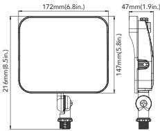
15W&27W(Knuckle Mount)
