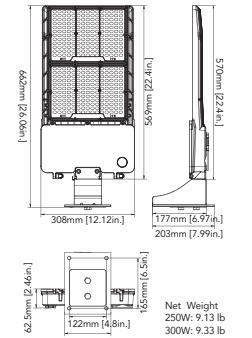
250W/300W (Wall Mount)
